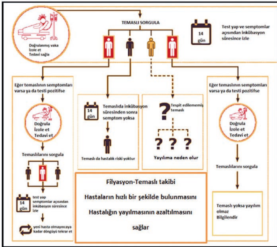
Resim-4: Filyasyonun şematik gösterimi
